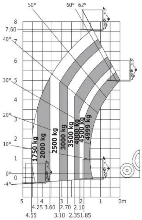
Ruw terrein lastendiagram (EN1459B) 500mm lastzwaartepunt
