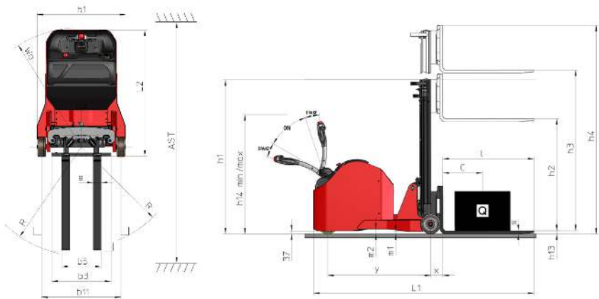
ES-C 720 - Tekening met afmetingen
