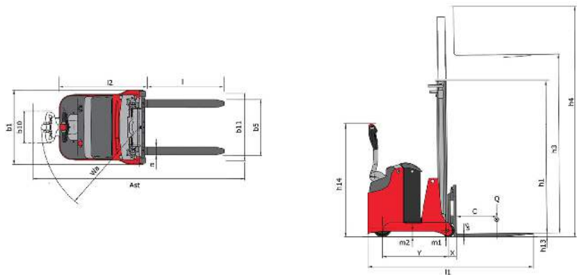
ES-C 510 - Tekening met afmetingen
