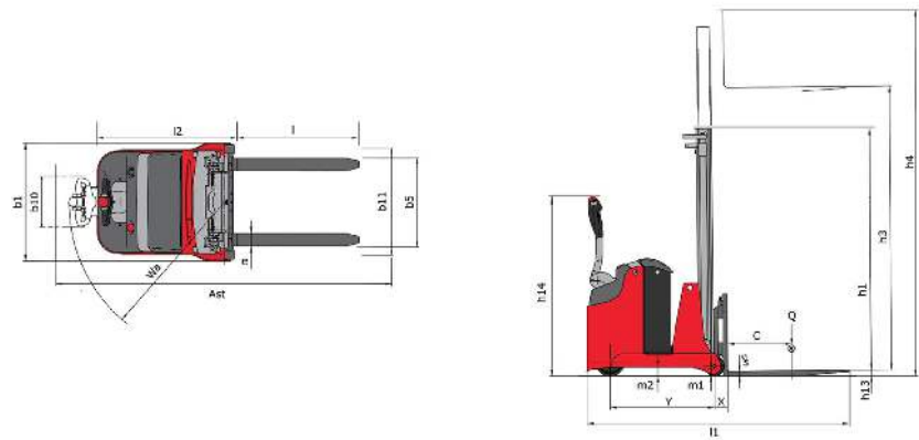
ES-C 507 - Tekening met afmetingen
