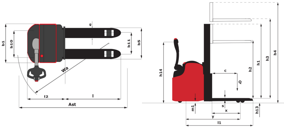
ES 730 - Tekening met afmetingen
