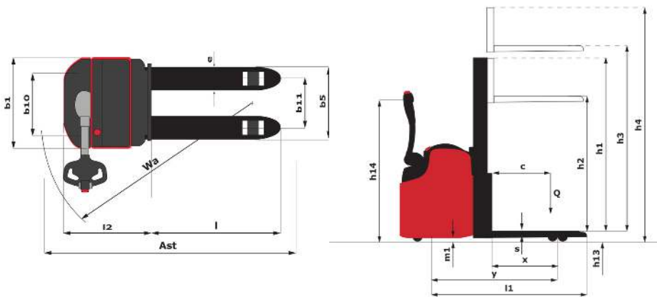
ES 720 - Tekening met afmetingen
