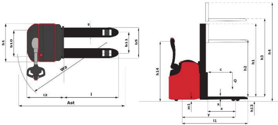
ES 614 LI - Tekening met afmetingen
