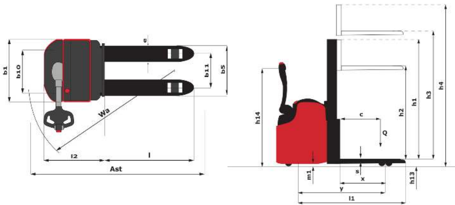
ES 612 LI - Tekening met afmetingen
