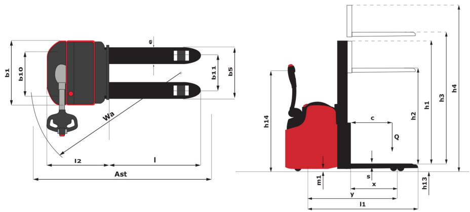
ES 414 - Tekening met afmetingen
