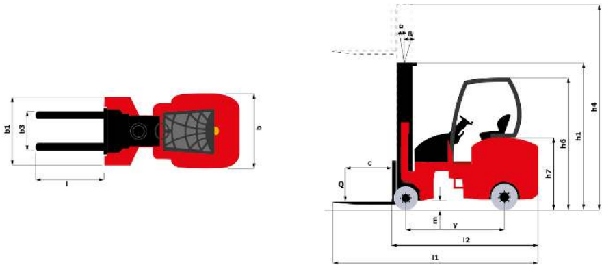
EMA II 20 HD-1 - Tekening met afmetingen
