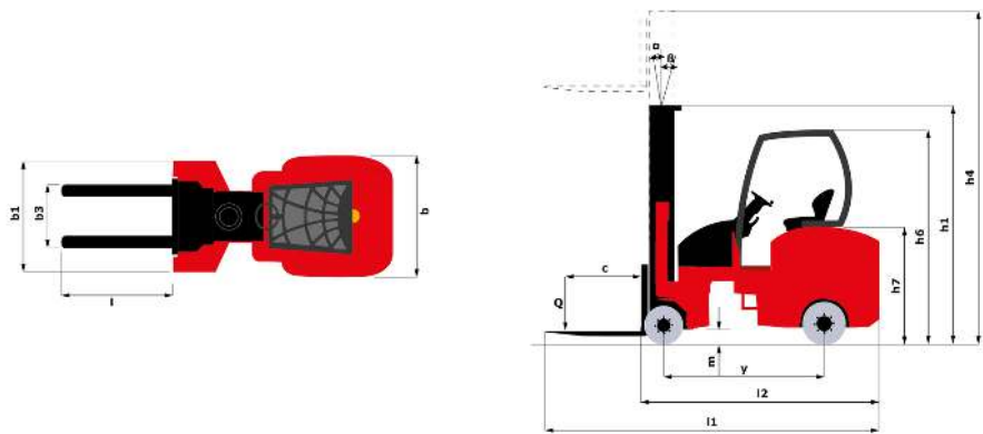
EMA II 18 HL-2 - Tekening met afmetingen
