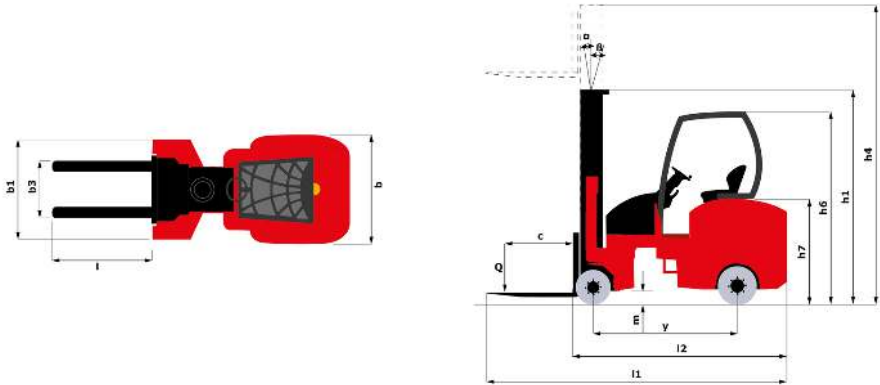
EMA II 18 HL-1 - Tekening met afmetingen
