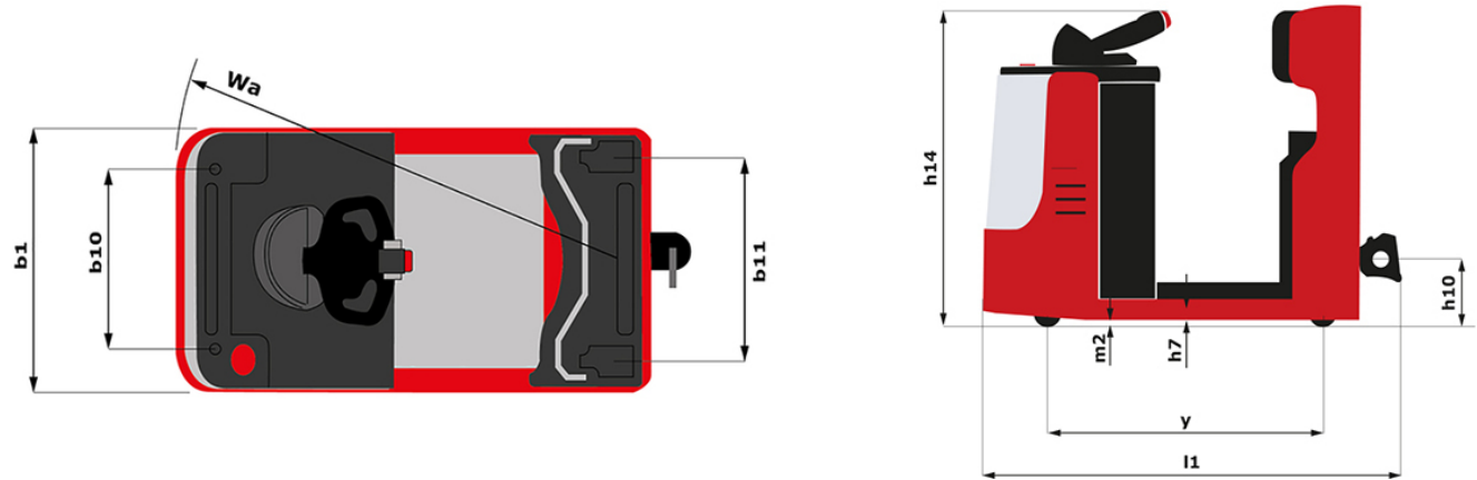
CT 30 - Tekening met afmetingen
