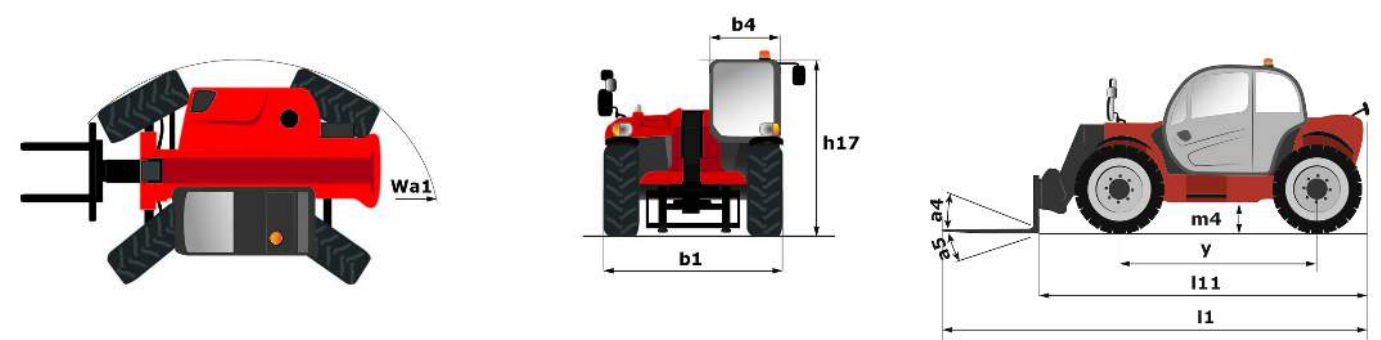
MT 930 H - Tekening met afmetingen
