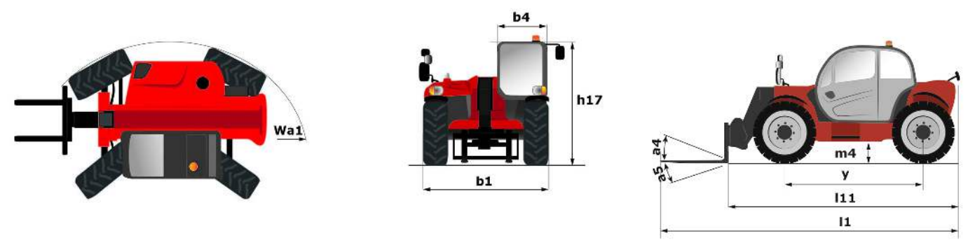
MT 730 H - Tekening met afmetingen
