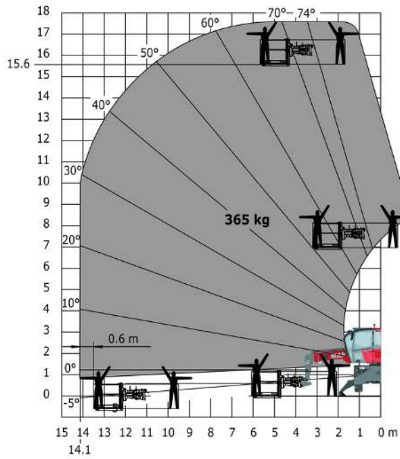
Rotatie op verlaagde stabilisatoren met 365 kg platform
