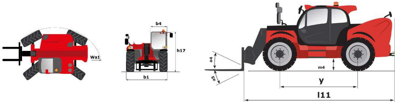
MLT 961-160 V+ L - Tekening met afmetingen
