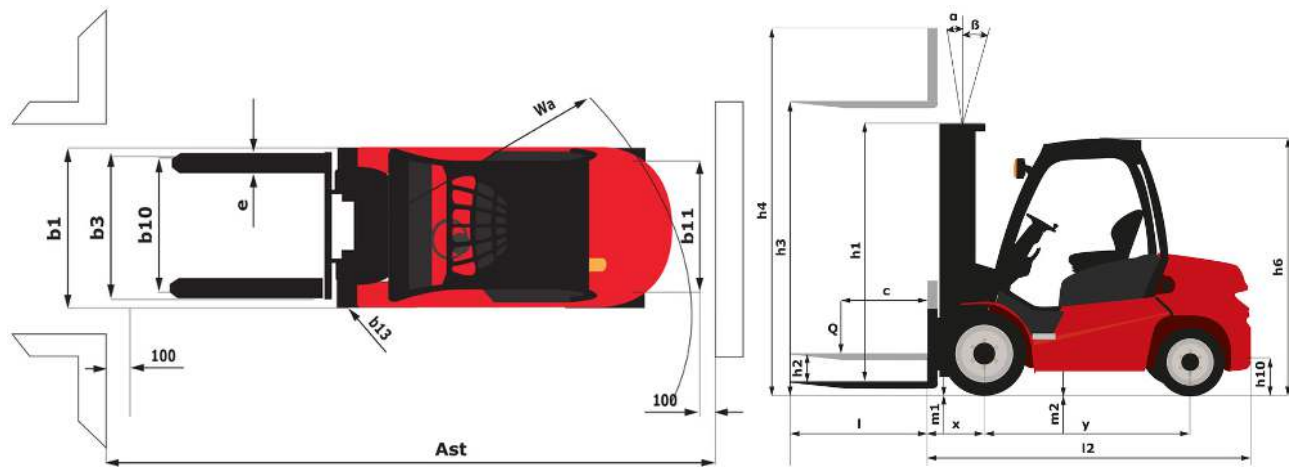
MI 55 G ST5 - Tekening met afmetingen
