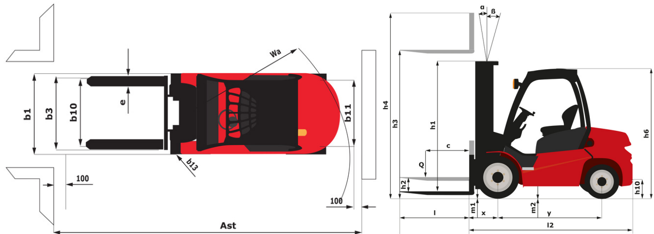
MI 35 D ST5 - Tekening met afmetingen
