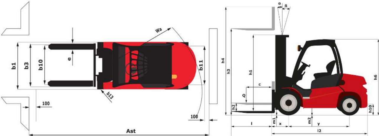
MI 25 D ST5 - Tekening met afmetingen
