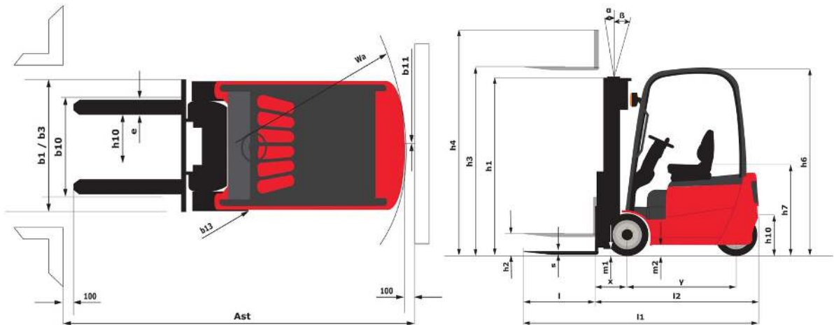
ME 440 - Tekening met afmetingen
