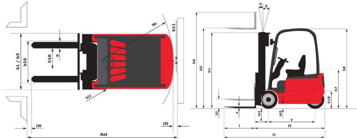
ME 318 - Tekening met afmetingen
