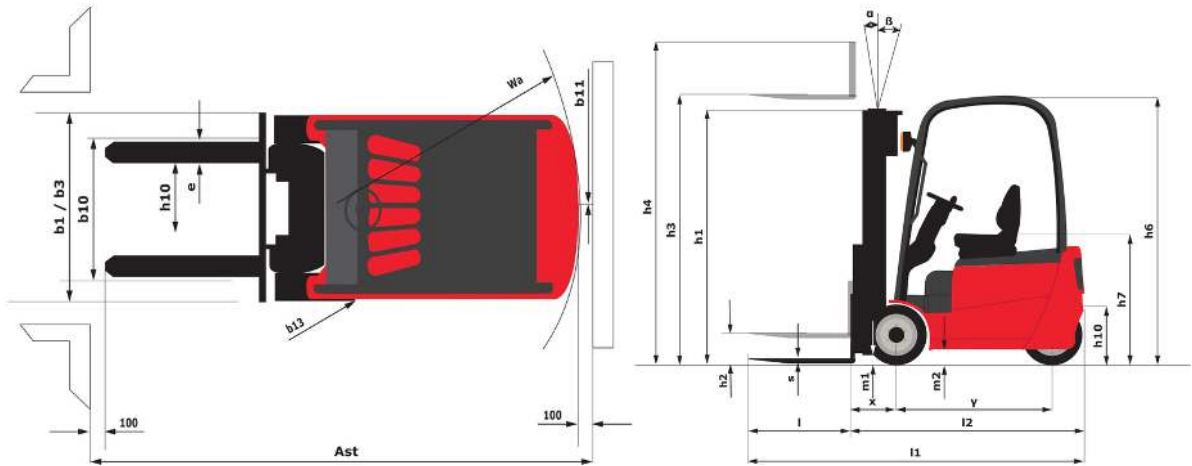
ME 315 - Tekening met afmetingen
