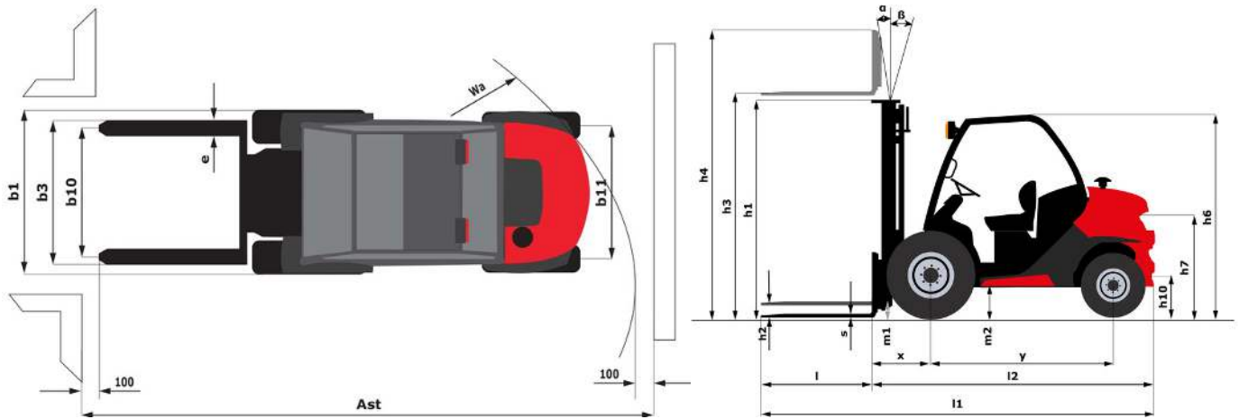
MC 25-2 ST5 - Tekening met afmetingen
