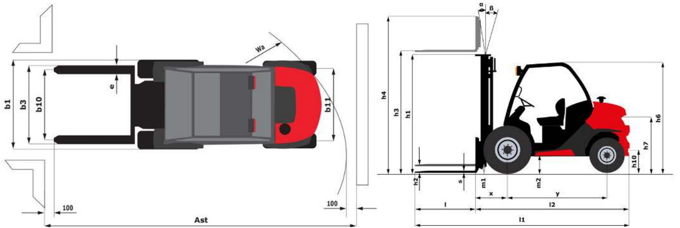
MC 18-4 ST5 - Tekening met afmetingen
