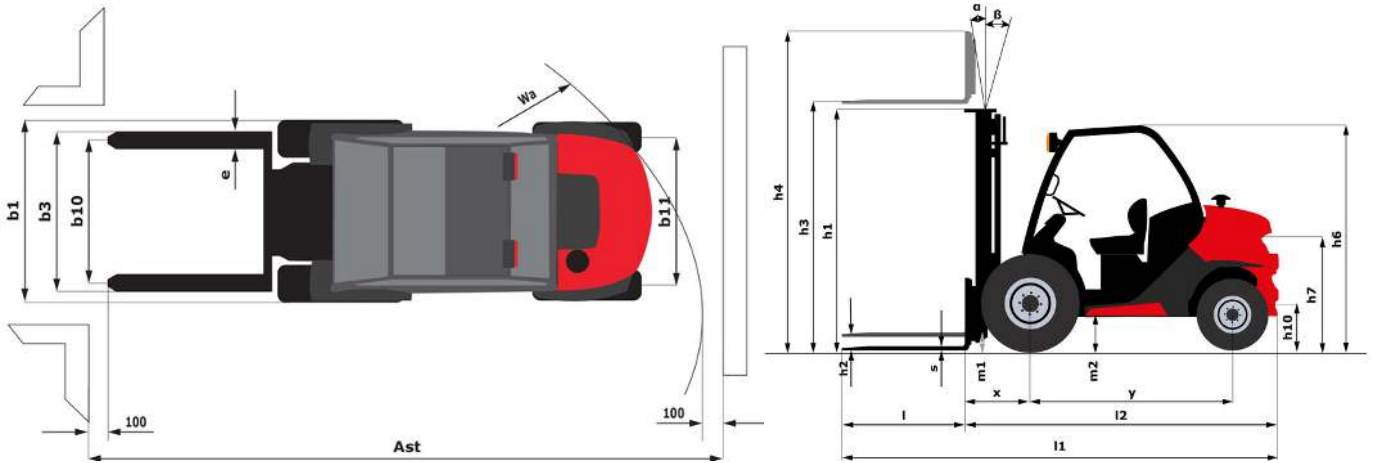
MC 18-2 ST5 - Tekening met afmetingen
