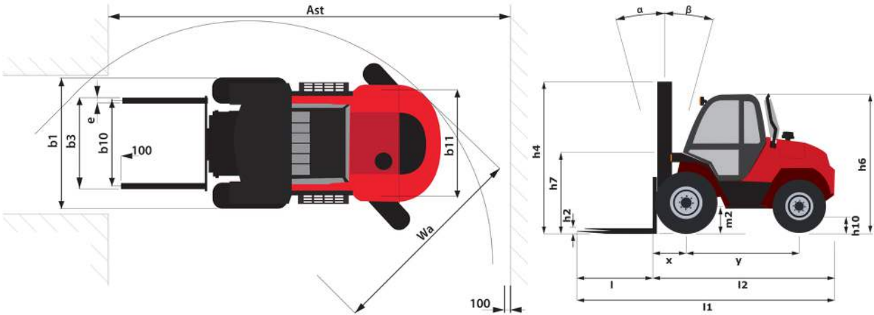
M 70-2 H D ST5 - Tekening met afmetingen
