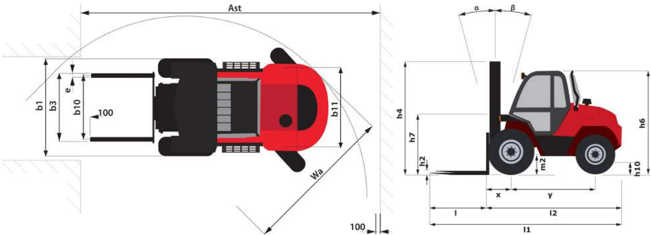
M 30-2 D ST5 - Tekening met afmetingen
