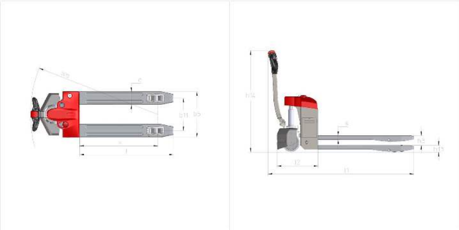
EP 15 Lithium Easy - Tekening met afmetingen
