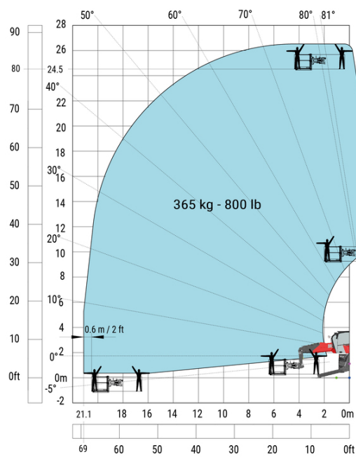
Rotatie op verlaagde stabilisatoren met 365 kg platform
